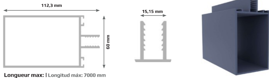
2 Poutre Viga
