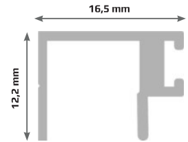
5 Bande d'étanchéité Sellado de puerta
