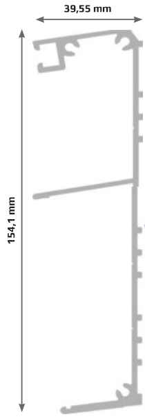
1 Profil mural Perfil de pared
