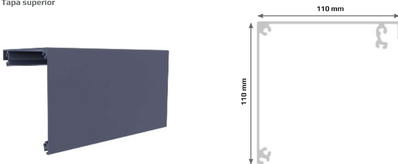
1 Capot supérieur Tapa superior
