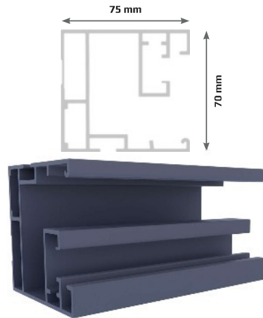
2 Guidage latéral Guía lateral
