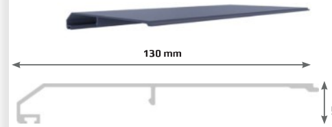
6 Liste de tirage Lista de tirador
