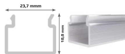
19115 8 Rail supérieur Riel superior
