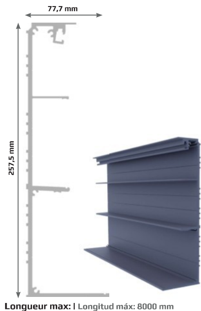
1 Profil mural Perfil de pared
