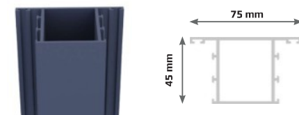
1770 4 Liste intermédiaire Listón intermedio
