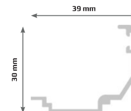
12 Profil pour encadrement de panneau Perfil para marco de panel
