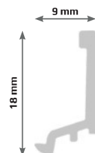
9 Profil pour barrette de verre double Perfil para listón de vidrio doble
