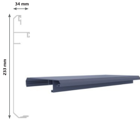
1 Capot supérieur Tapa superior
