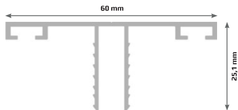
5 Cliquet supérieur Clic superior
