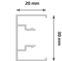
2 Profil de couverture Perfil de cubierta
