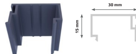
1795 7 Bandeau de verre Listón de vidrio
