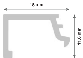
6 Profil pour barrette de verre simple Perfil para listón de vidrio sencillo
