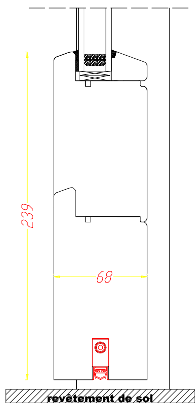
DDF-68 Porte d'entrée avec seuil tombant (sans seuil plat alu) - ouverte
