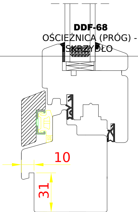
DDF-68 Découpe du dormant de l'extérieur
