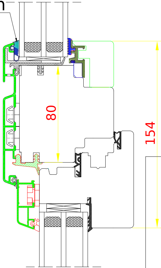
DDA-78 CLASSIC Fix - traverse - ouvrant
