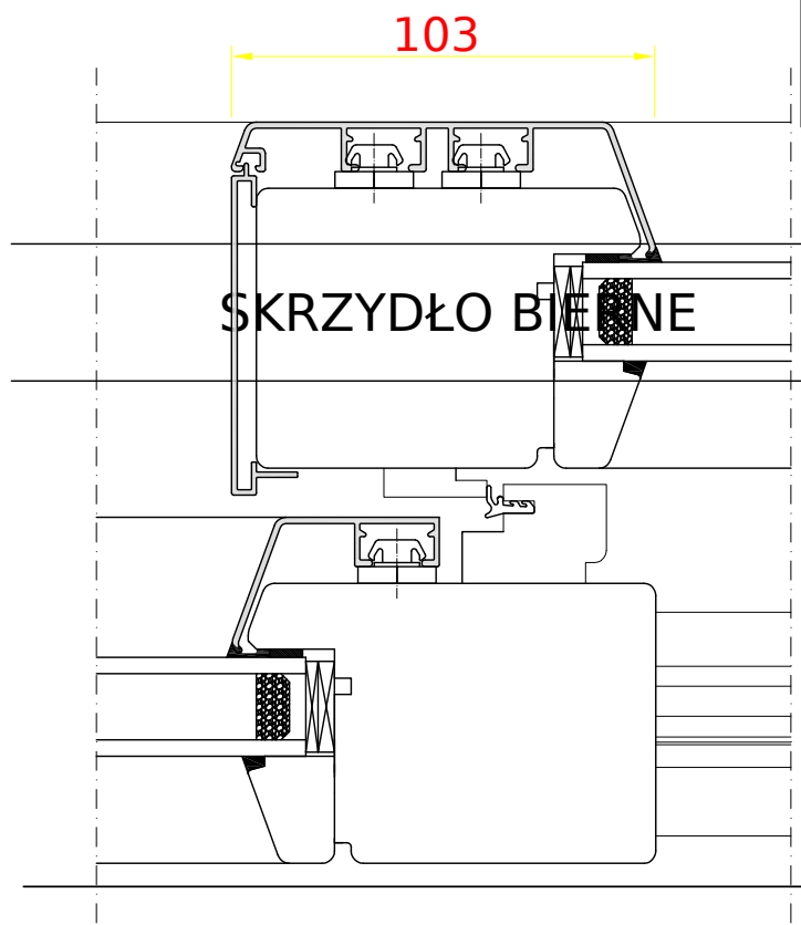
SKRZYDŁO DDF-68 AL Ouvrant - ouvrant
