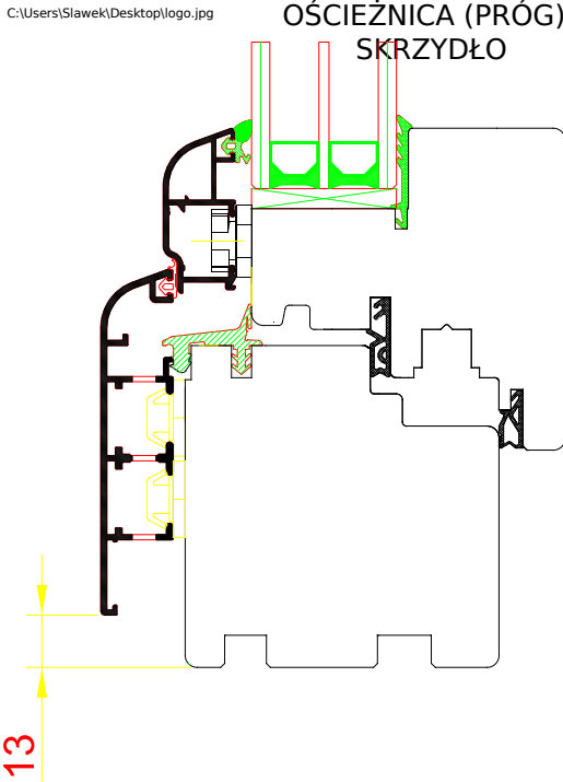
DDA-78 Softline Dormant (seuil) ouvrant
