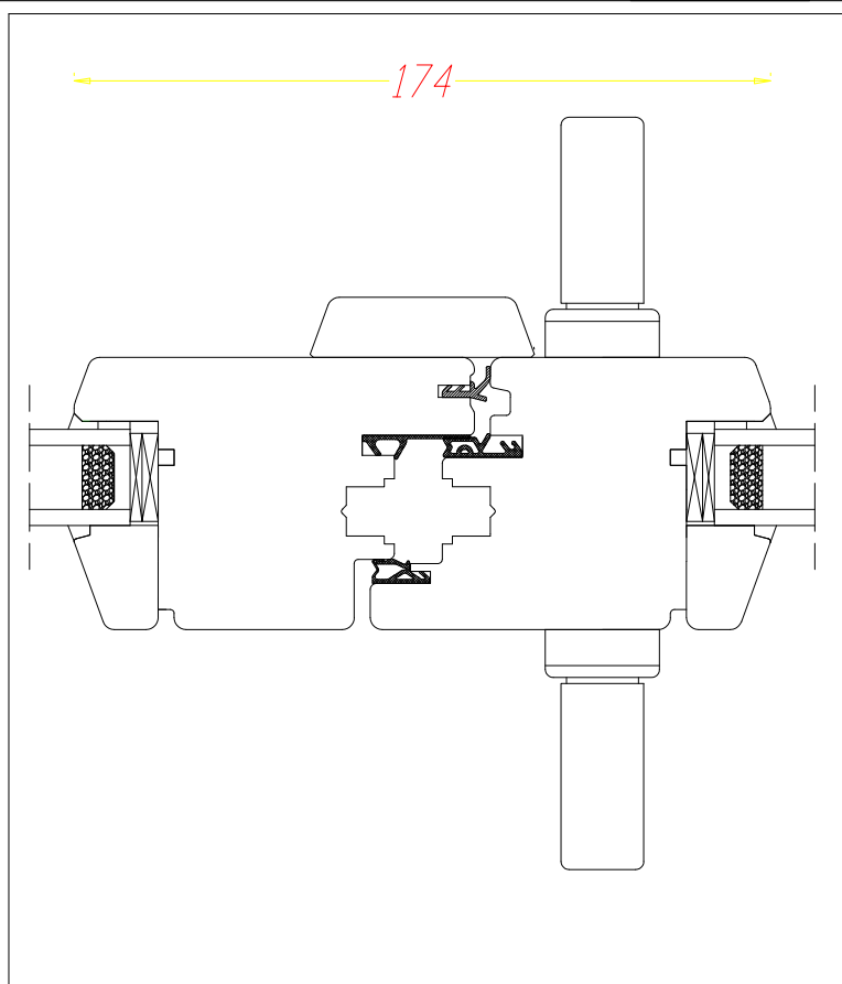
DDF-68 Porte fenêtre Double poignée avec serrure
